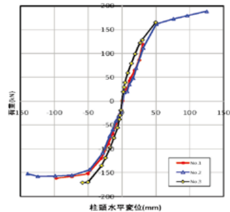
図-3 荷重-柱頭水平変位包絡線
