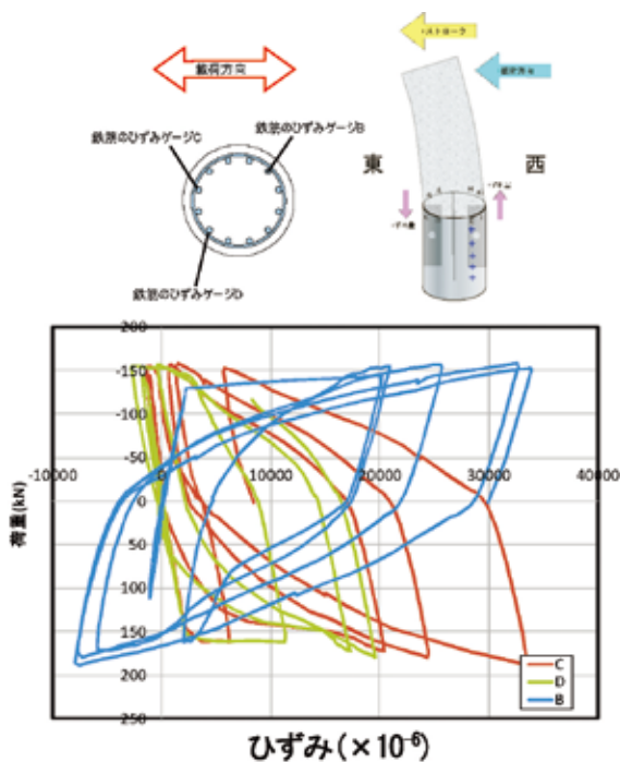
図-4 RC柱と鋼管継ぎ目の鉄筋のひずみ曲線
