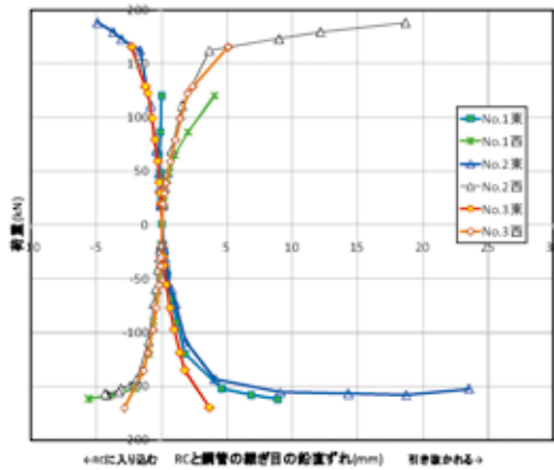
図-6 荷重-RCの鋼管からの抜け出し量の包絡線
