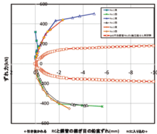
図-7 PBL 1孔あたりのせん断力-ずれ曲線
