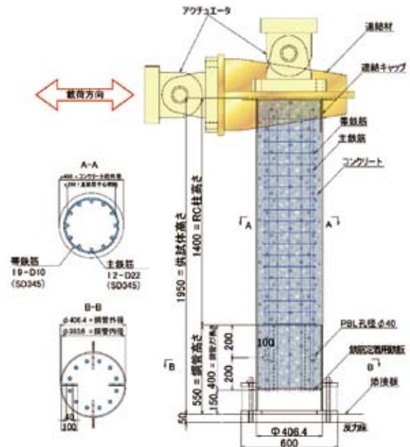
図-1 供試体形状
