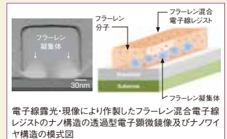
電子線露光・現像により作製したフラーレン混合電子線レジストのナノ構造の透過型電子顕微鏡像及びナノワイヤ構造の模式図
