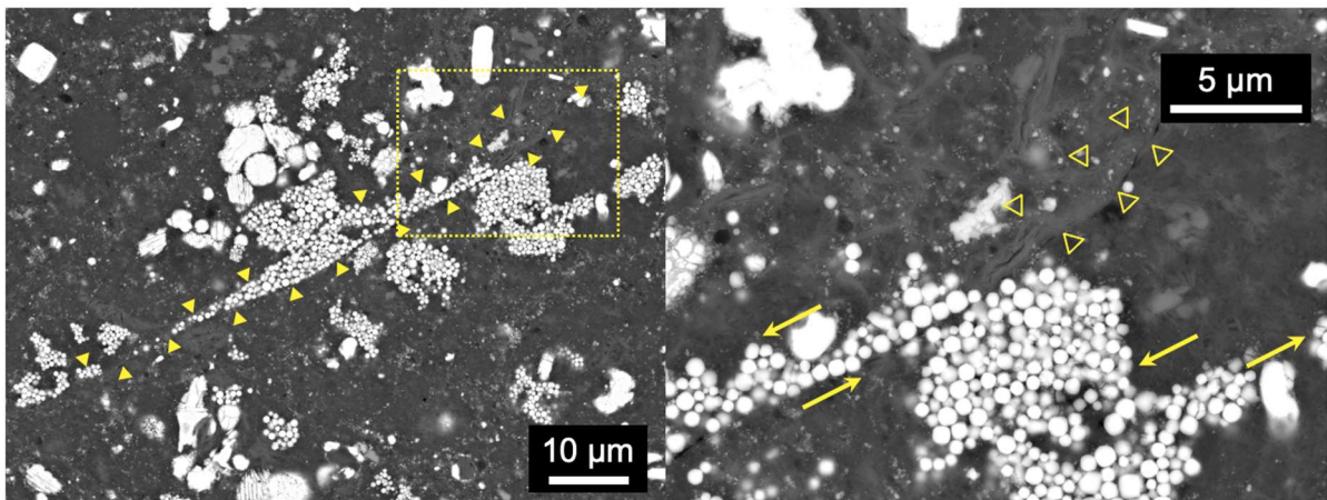
図2 リュウグウ粒子中に見られる断層組織の走査電子顕微鏡像。明るい粒子は酸化鉄(マグネタイト)。(左)球状の酸化鉄微粒子集合体(フランボイド)が断層によって引き伸ばされている。(三角矢印で示された領域)、(右)左図の点線で囲まれた領域の拡大像。断層に沿った粘土鉱物(三角矢印で示された領域)には、気泡や鉄-硫黄-酸素に富む微粒子などの熔融組織は認められない。矢印は断層のずれの方向を示す。
