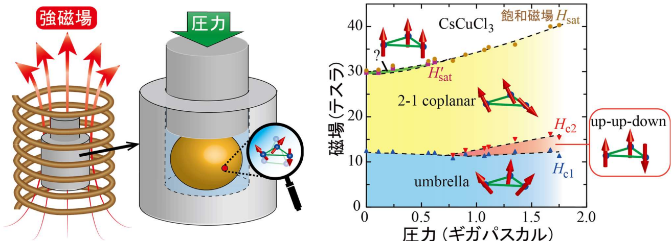
図1(左):強磁場高圧力下磁化測定装置の概略図。パルス強磁場・高圧力発生装置の内部に試料と磁化検出コイルの両方を配置することで強磁場・高圧力下における微弱な磁化検出に成功。(右)三角格子反強磁性体 \text{CsCuCl}_3 の磁場-圧力相図。飽和磁場は、圧力増加に伴い高磁場側に移動し、最高圧力 1.7 ギガパスカルで 40 テスラまで到達。
