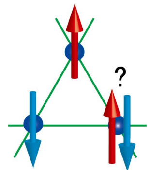
図2 スピンのフラストレーション。矢印の向きがスピンの向きを表す。
