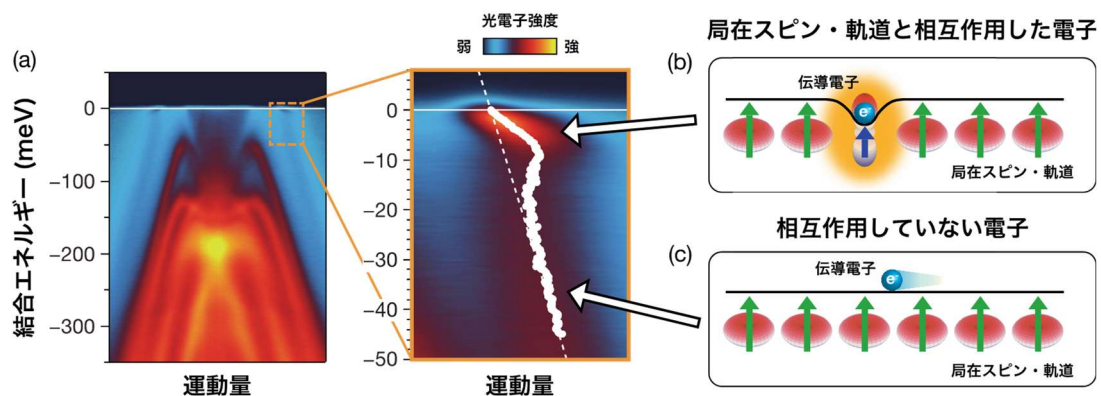
図1：(a) レーザー光電子分光で観測したセリウム・アンチモンの電子構造。相互作用で重くなった伝導電子(準粒子)に対応する電子構造の折れ曲がり観測されました。(b, c) 本研究で
