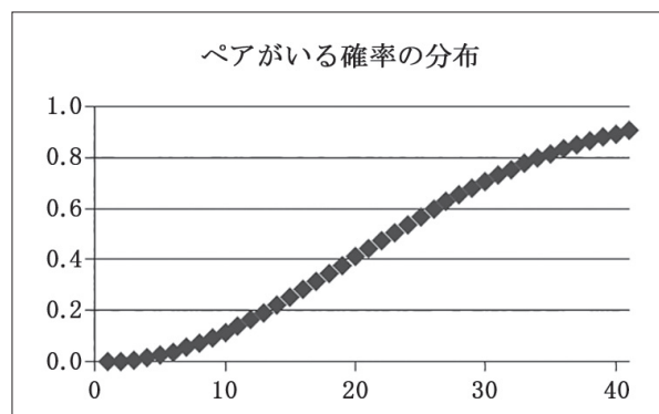
図1. 確率の分布
